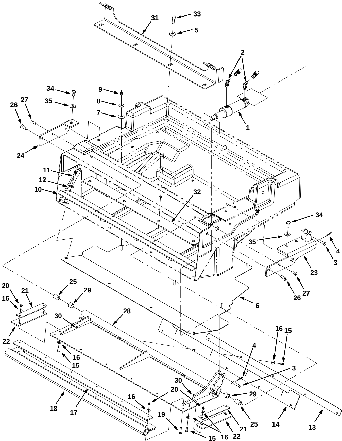
Fig. 41 – Hopper Door Group (000000-003061)
