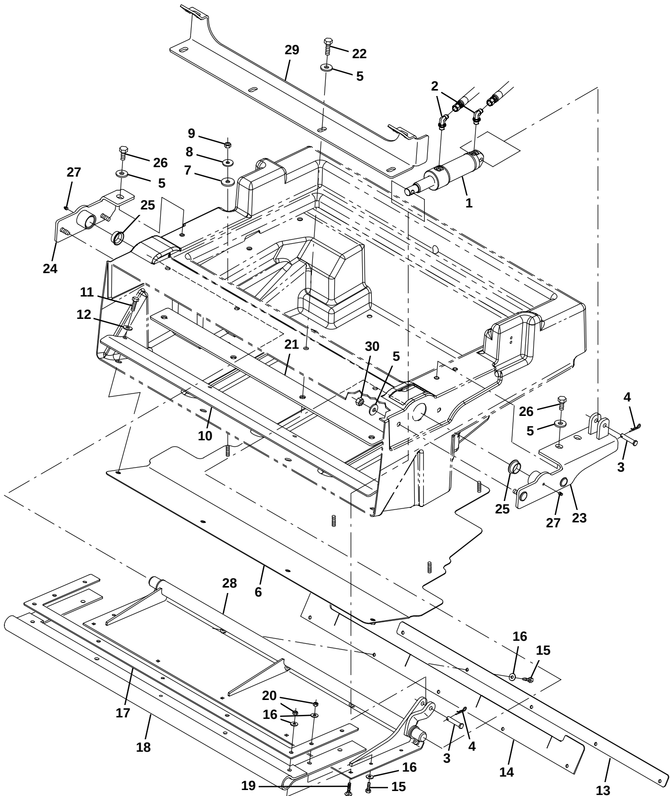
Fig. 42 – Hopper Door Group (003062– )
