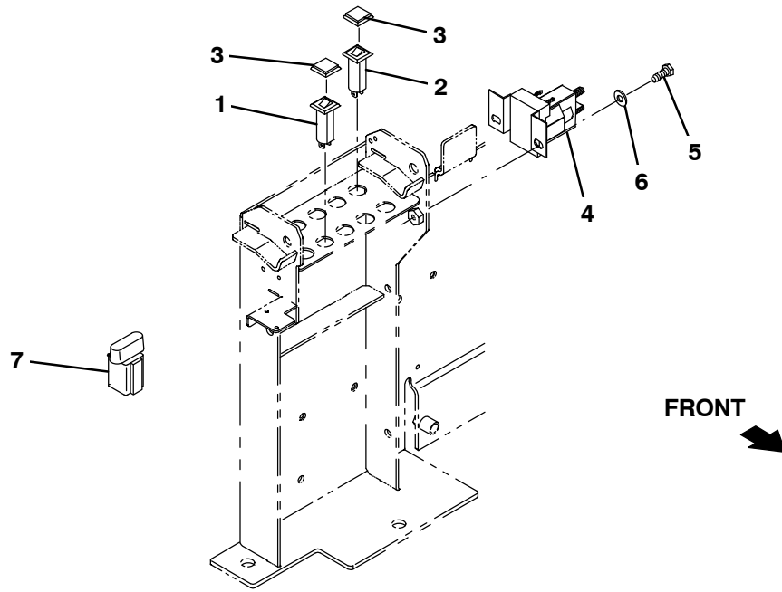
Fig. 16 – ES Electrical Group
