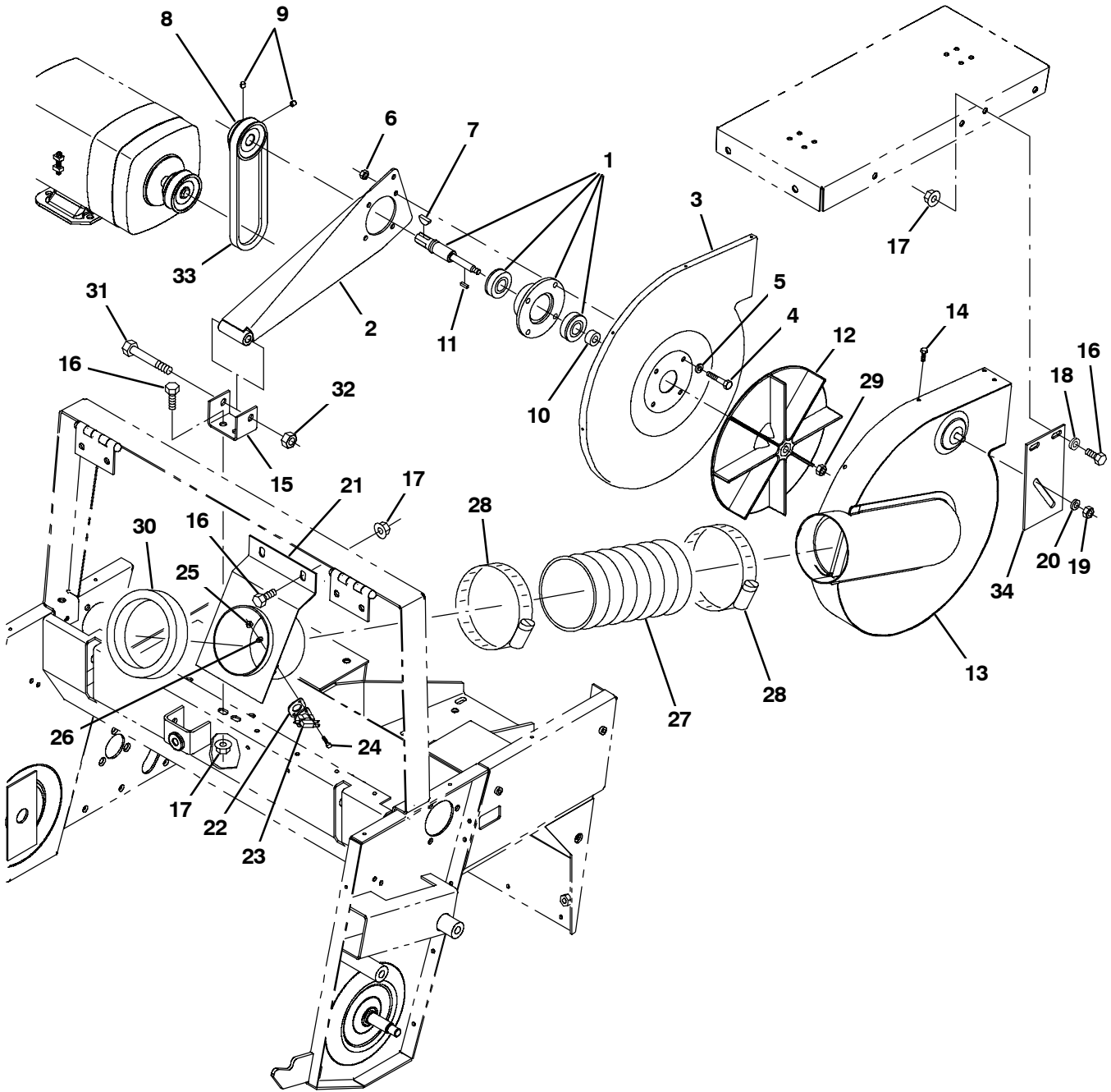
Fig. 14 - Vacuum Fan Group
