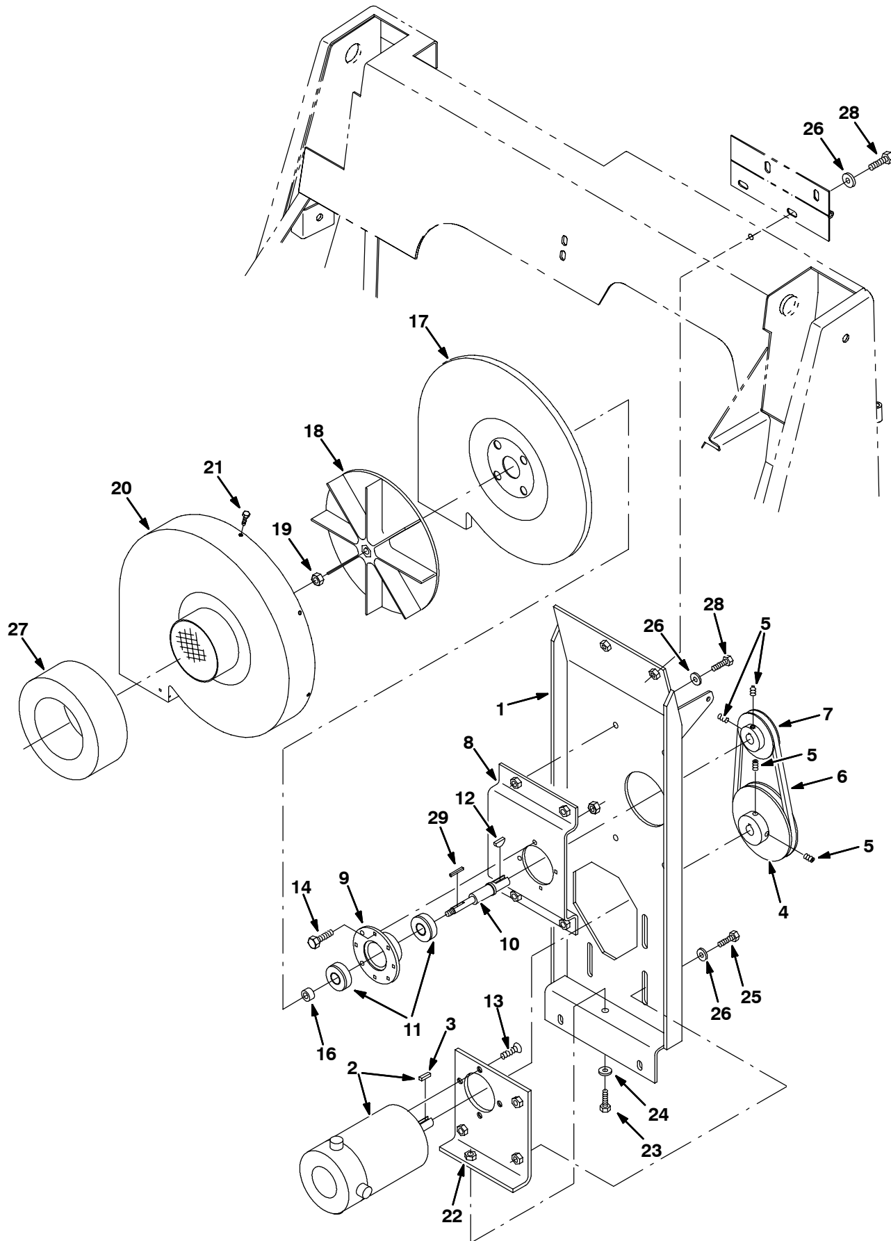
Fig. 44 - Sweeper Vacuum Fan Group
