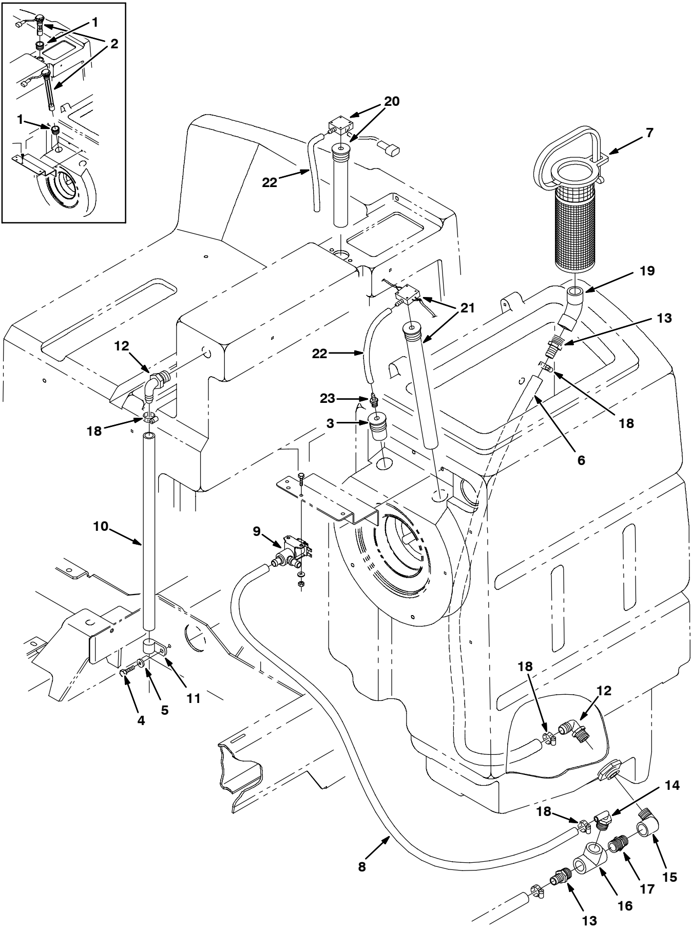
Fig. 4 - ES Tanks Group (000000- 001453)
