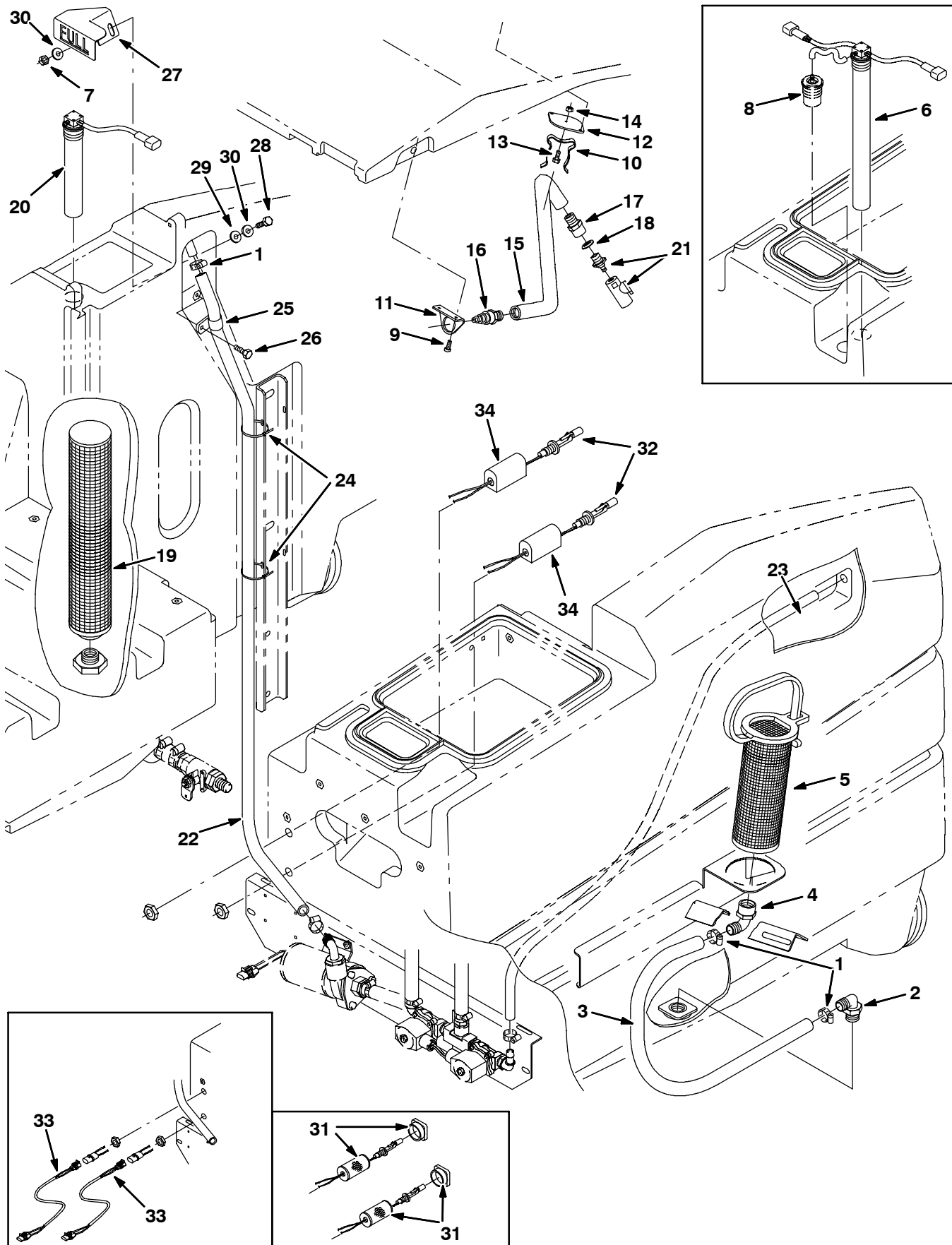
Fig. 44 - ES Tank Group
