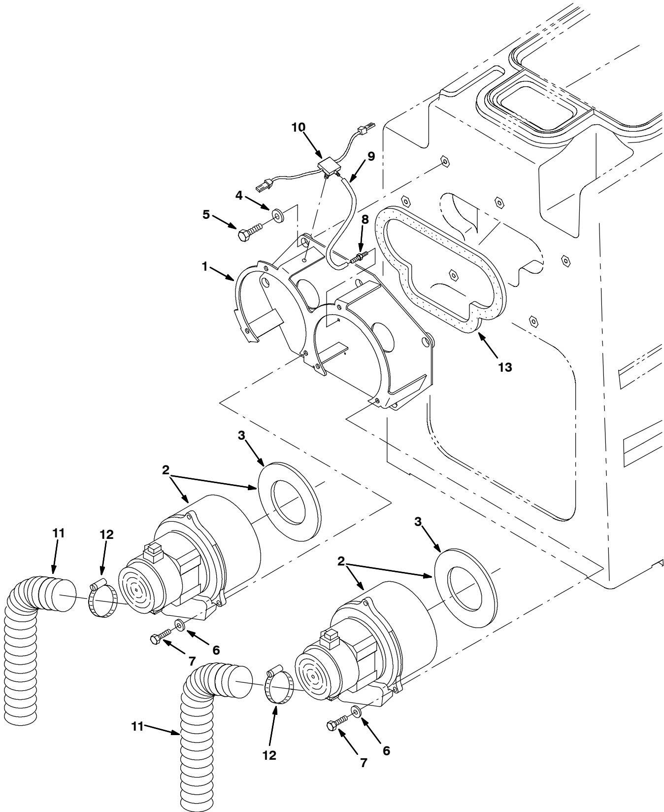
Fig. 21 - Vacuum Fan Group
