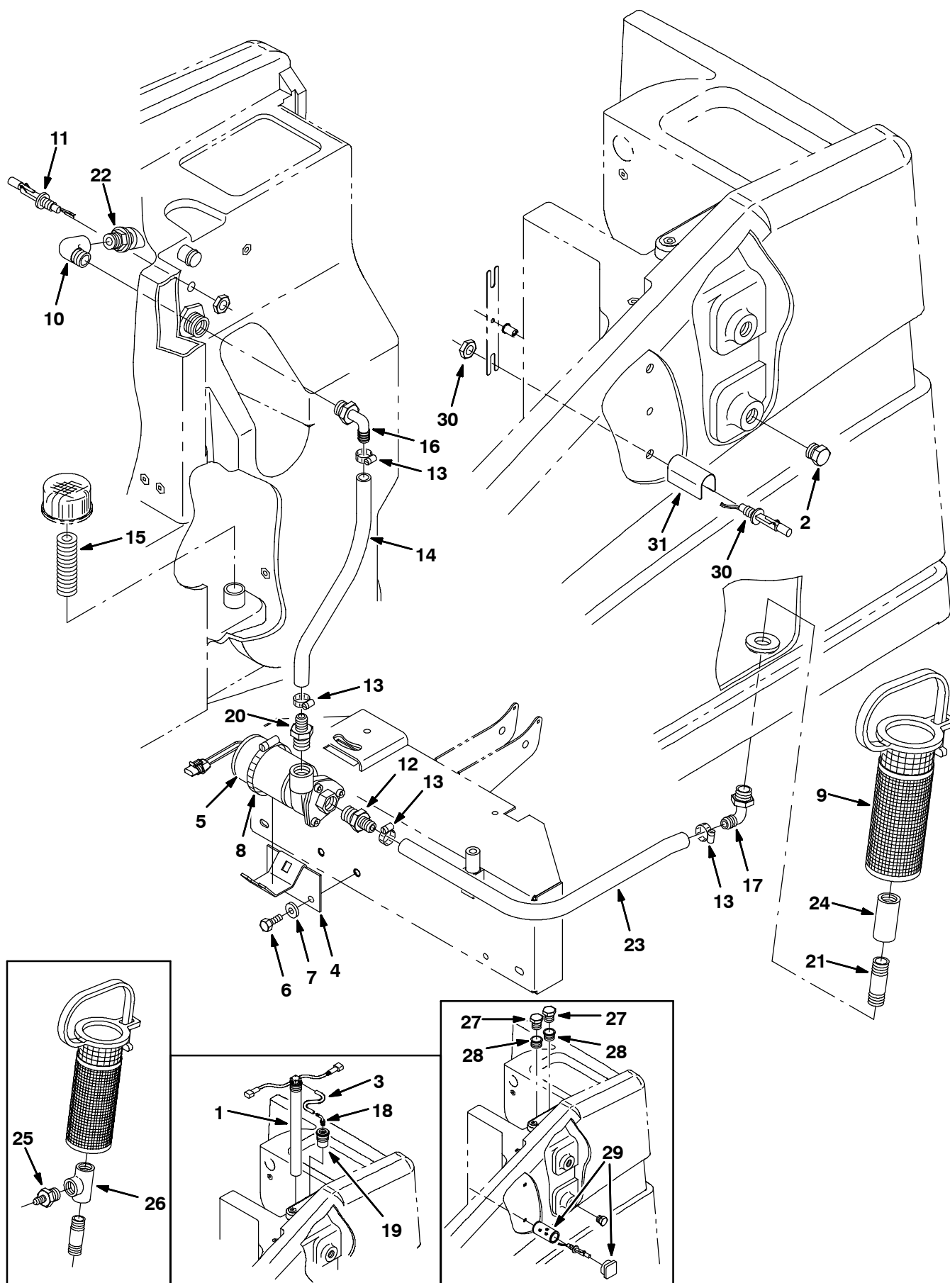
Fig. 10 - ES Pump Group (007062- )
