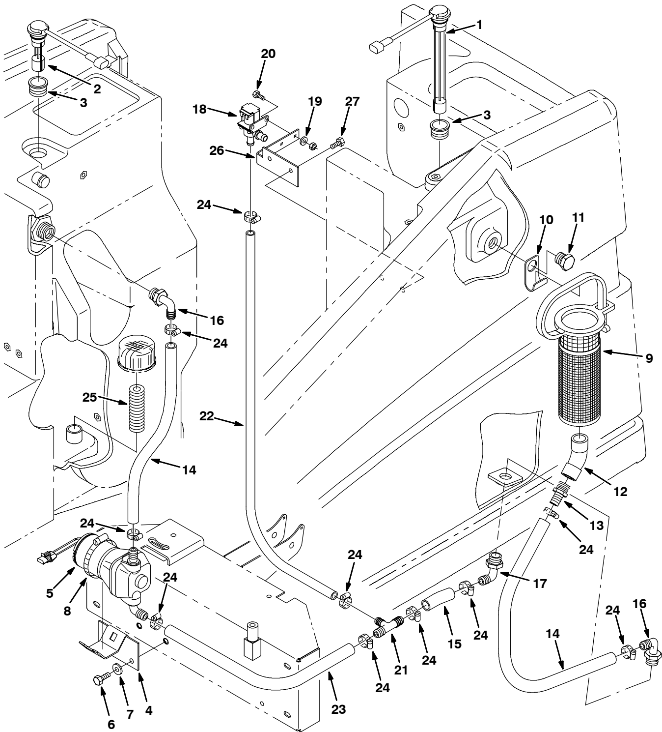
Fig. 8 - ES Pump Group (006140-006497)
