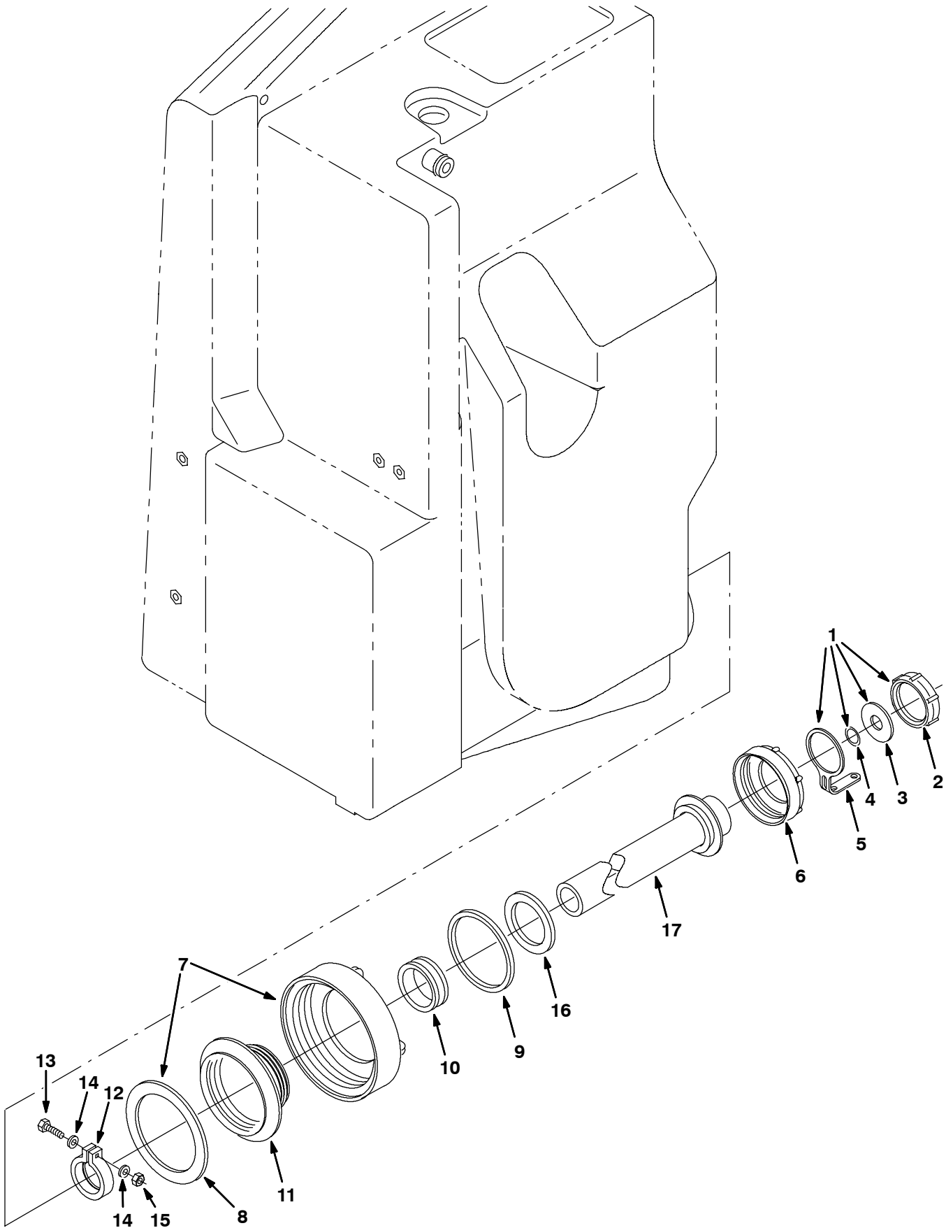
Fig. 12 - ES Drain Group
