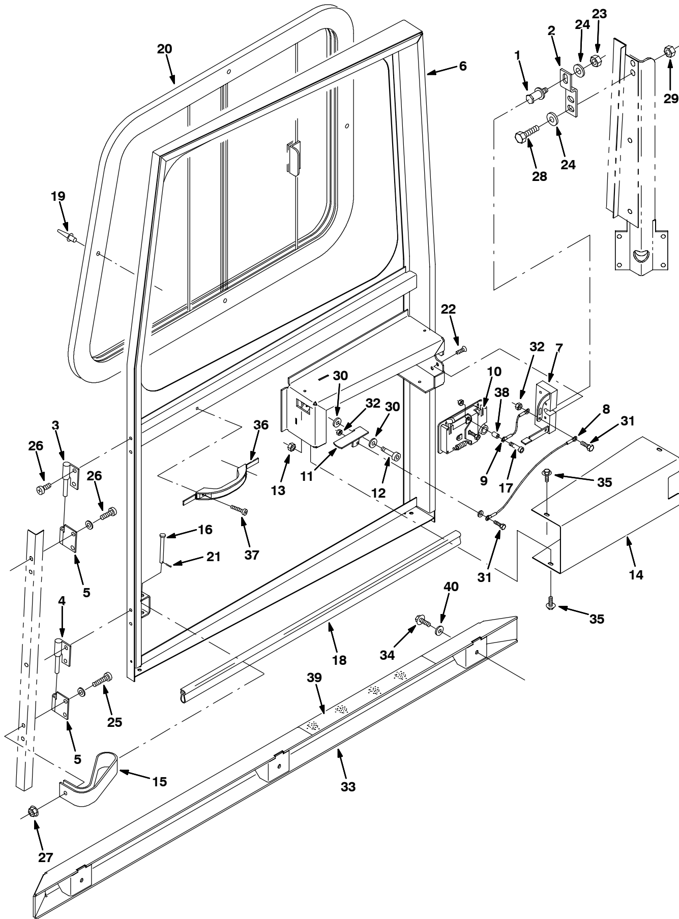
Fig. 15 - Cab Door Group
