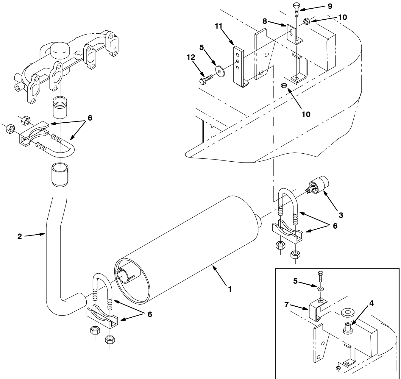
Fig. 23 - Muffler Group
