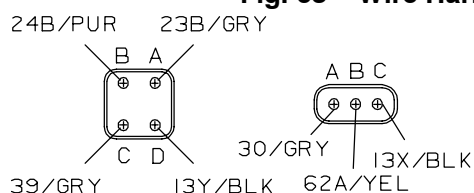
VIEW A-A
